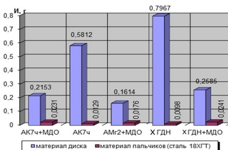
Рисунок 1 – Результаты испытаний пар трения «диск - пальчики»
